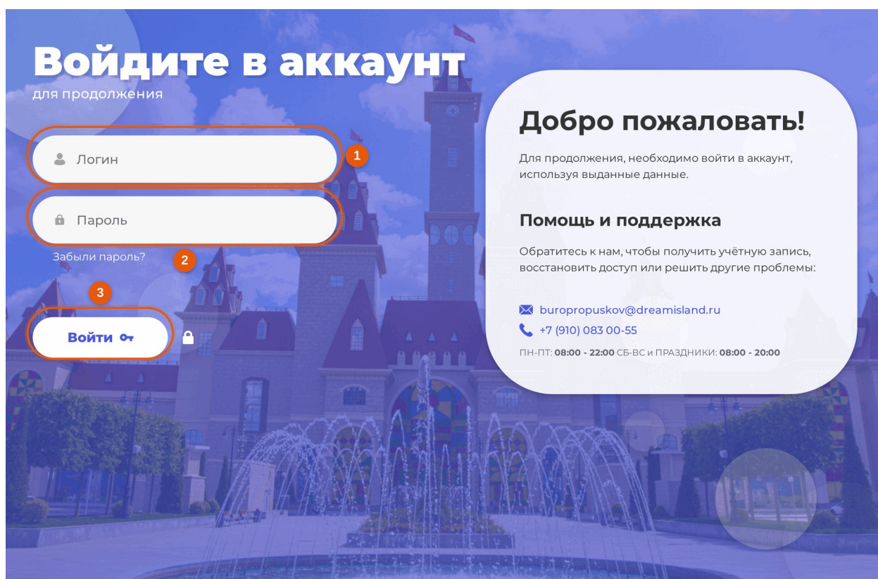
Рисунок 3.1 — Страница входа
