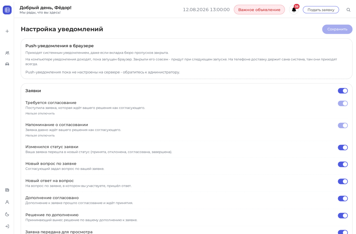
Рисунок 9.7 — Настройка уведомлений
